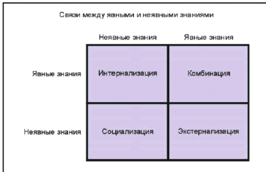
Рисунок 4 - Модель SECI
