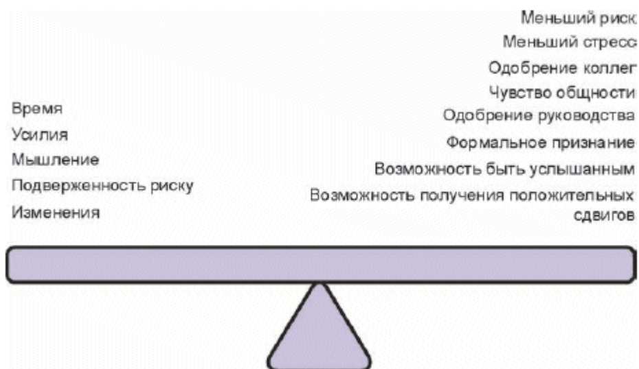
Рисунок 29 - Персональный баланс
